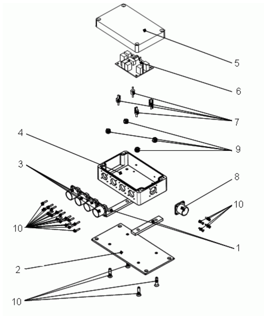
Рис. 9. Схема деления БОСДТ – 240 на части Fig. 9. БОСДТ-240 assembly
