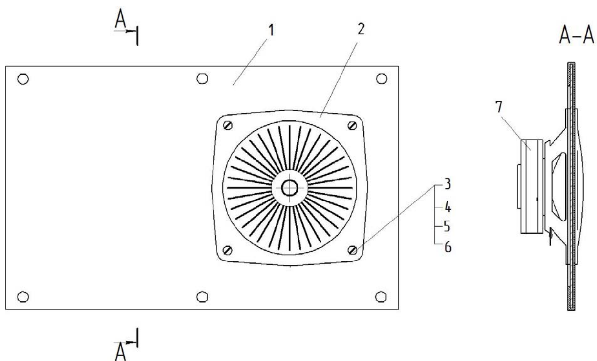
95-7 Панель 749-95-157СП Panel
