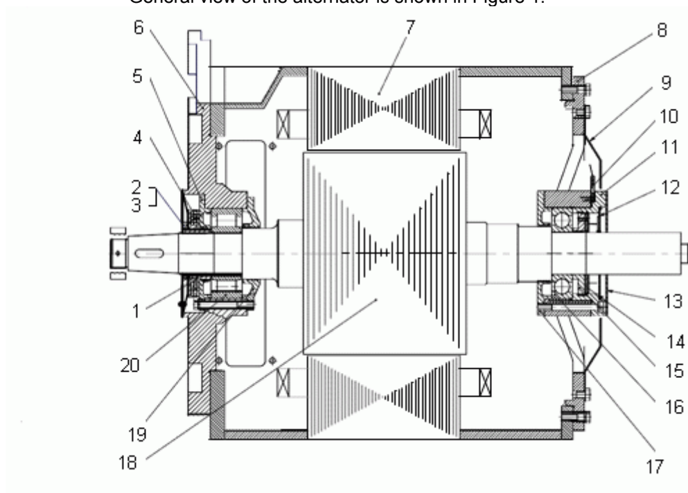
Рис. 1. Общий вид генератора ИГ – 250:
