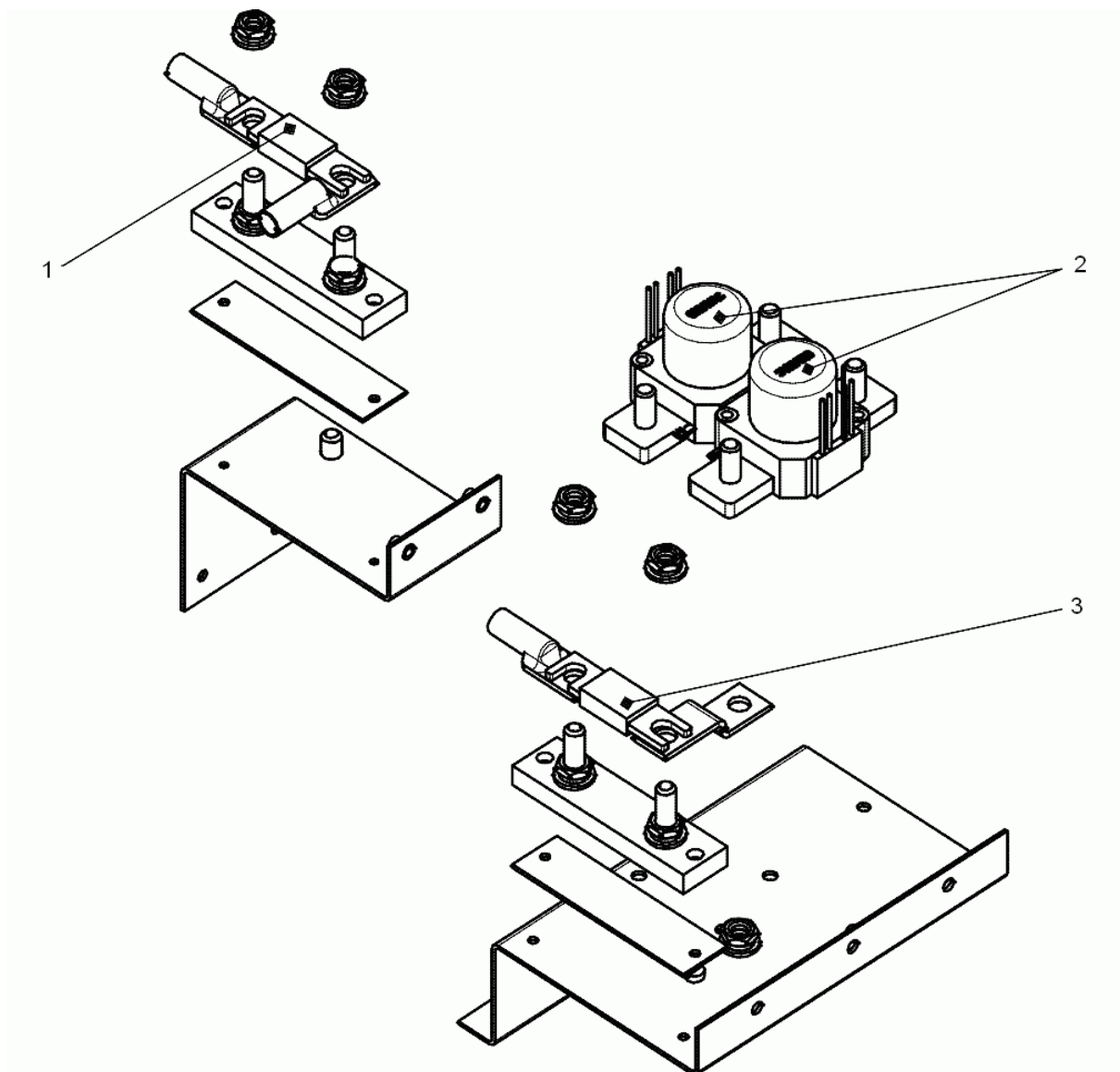
Рис. 6. Схема деления контакторов в сборе на части Fig. 6. Contactor assembly
