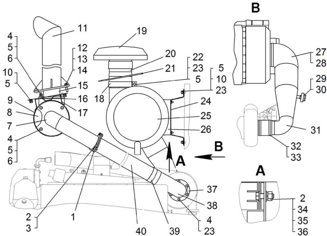
05-1 Система воздухопитания и выпуска Air inlet and outlet system
