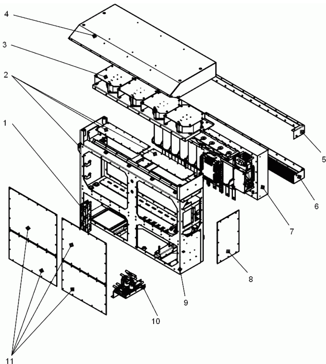
Рис. 2. Схема деления КТЭП-400 на части:
