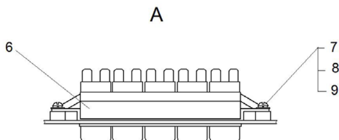
95-6 Панель 749-95-155СП Panel
