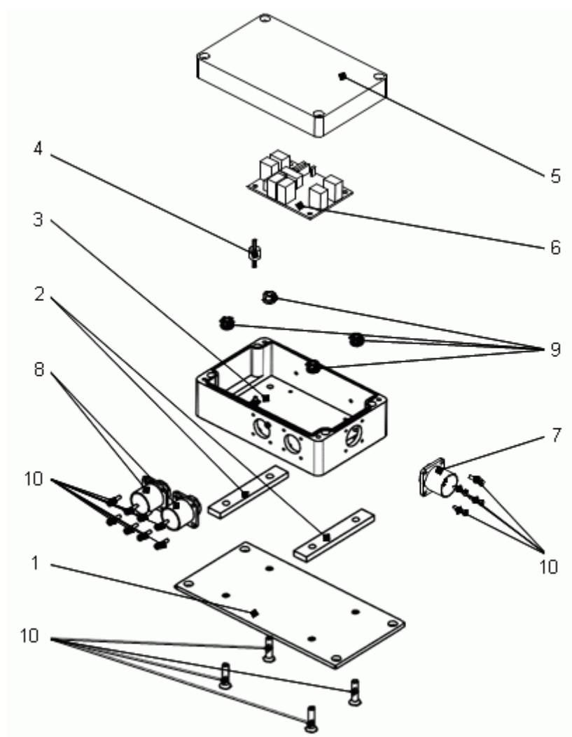
Рис. 10. Схема деления БОСДТ - 250 на части Fig. 10. БОСДТ-250 assembly
