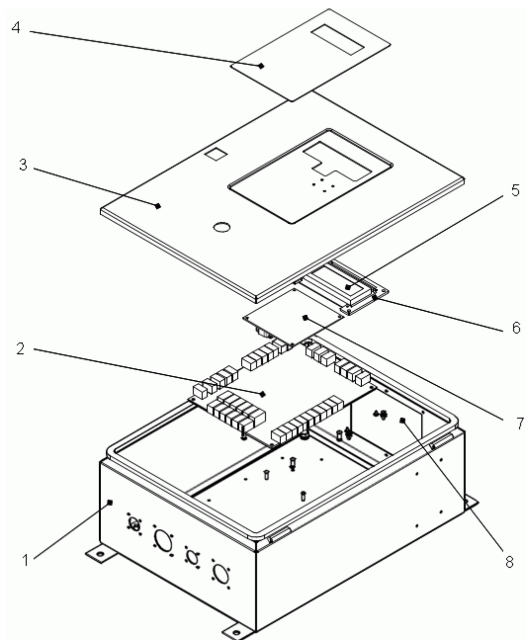
Рис. 8. Схема деления БМ-400 на части Fig. 8. БМ-400 assembly
