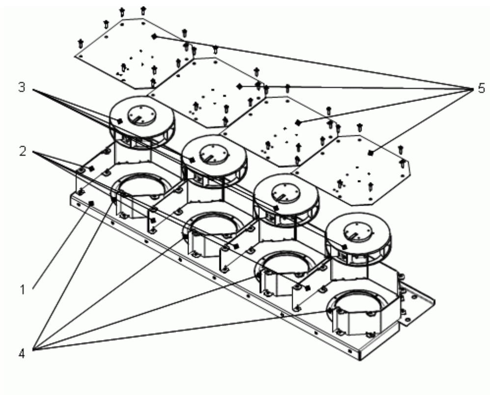
Рис. 4. Схема деления блока вентиляторов на части Fig. 4. Fan unit assembly
