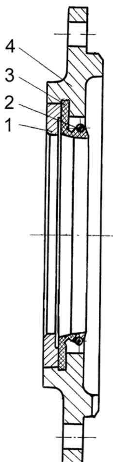
50-4 Крышка 748-50-123СП Cover
