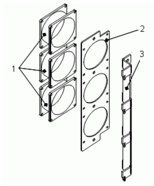
Рис. 5. Схема деления блока малых вентиляторов на части Fig. 5. Small fan unit assembly
