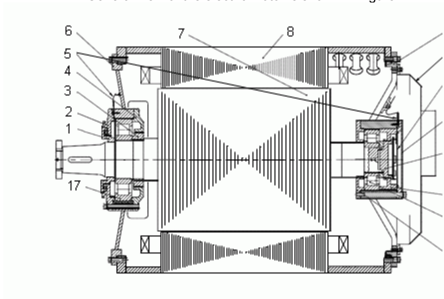
Рис. 1. Общий вид электродвигателя ИД – 240:
