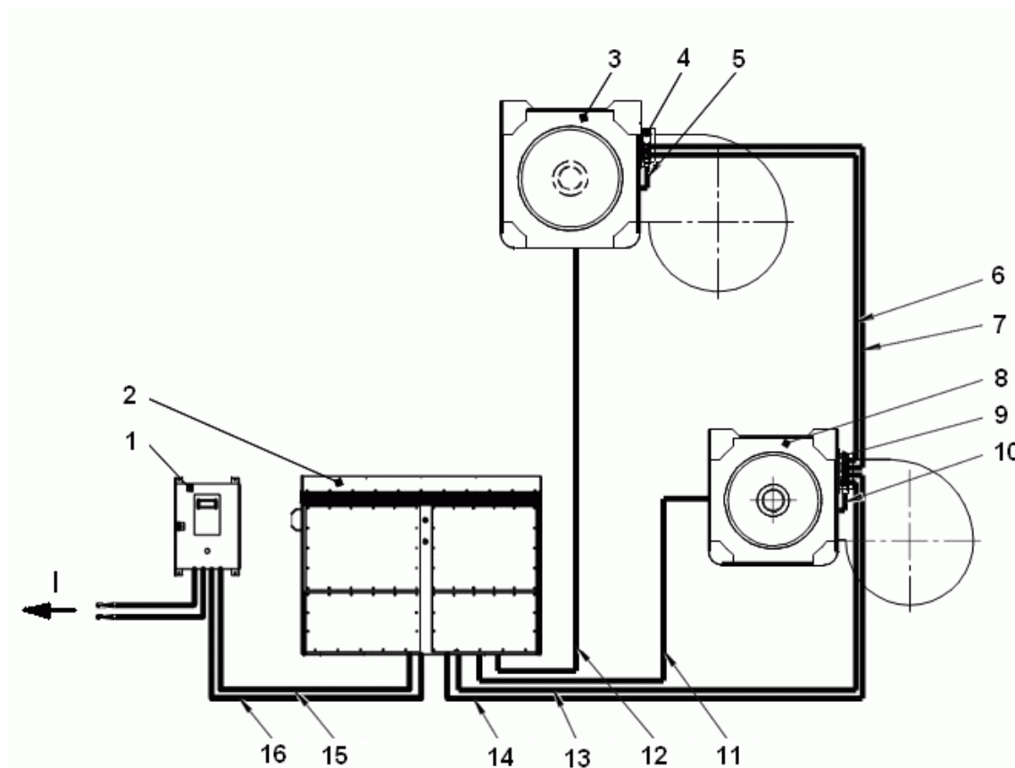
Рис.1. Схема деления КТЭП-400 на части
